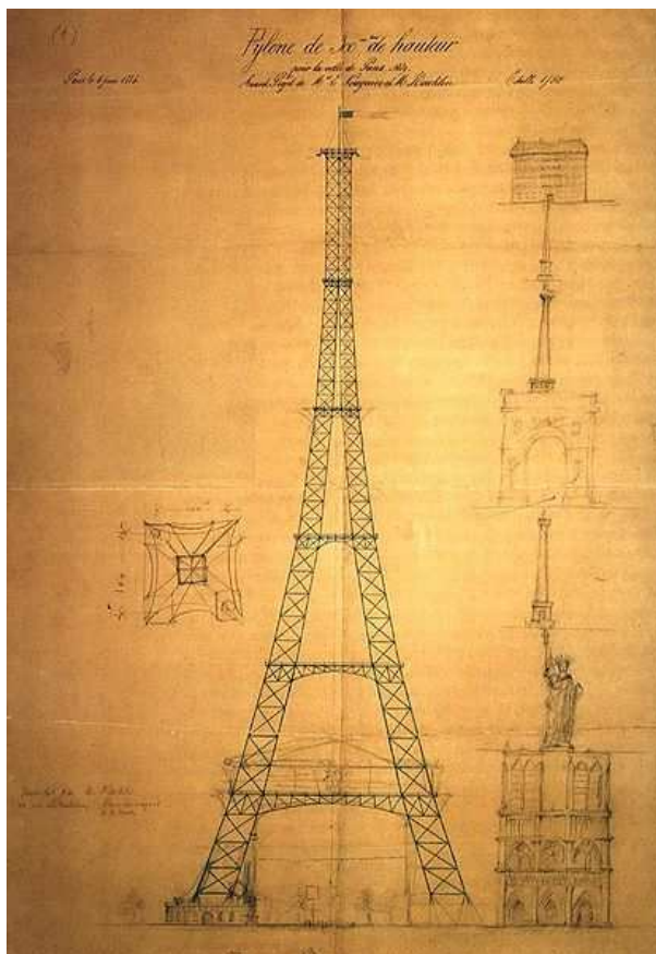
Primer esquema de la Torre Eiffel, de Emile Nouguier y Maurice Koechlin (1884). Fuente: http://moleskinearquitectonico.blogspot.com.es/
